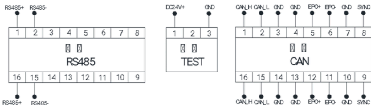
Rysunek 7. Wejścia sterownicze RJ45
