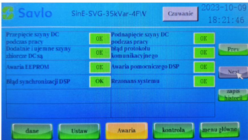
Rysunek 29. Zakładka awaria
