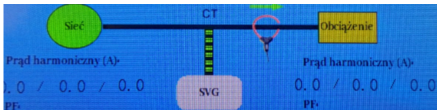
Rysunek 18. Ekran główny kompensatora przy przekładnikach od strony obciążenia/instalacji
